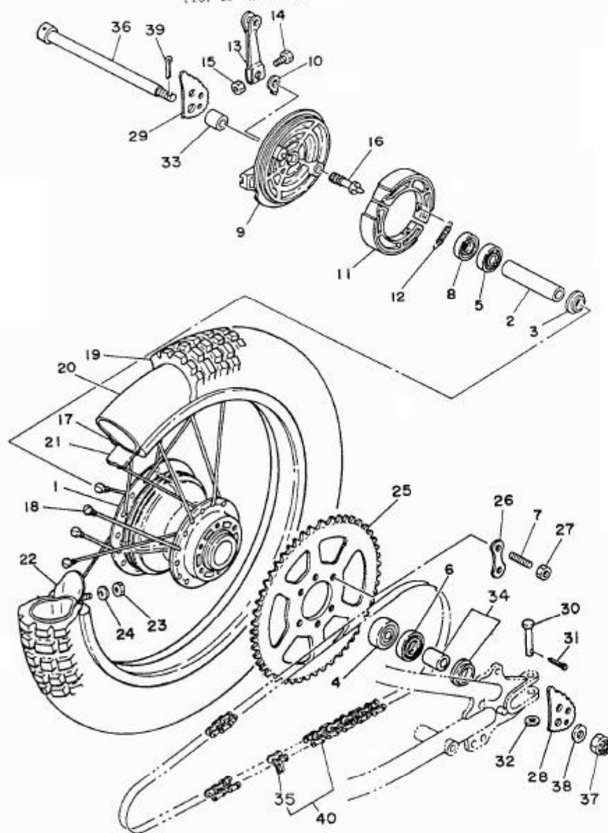
FIG. 28 RODA TRASEIRA
