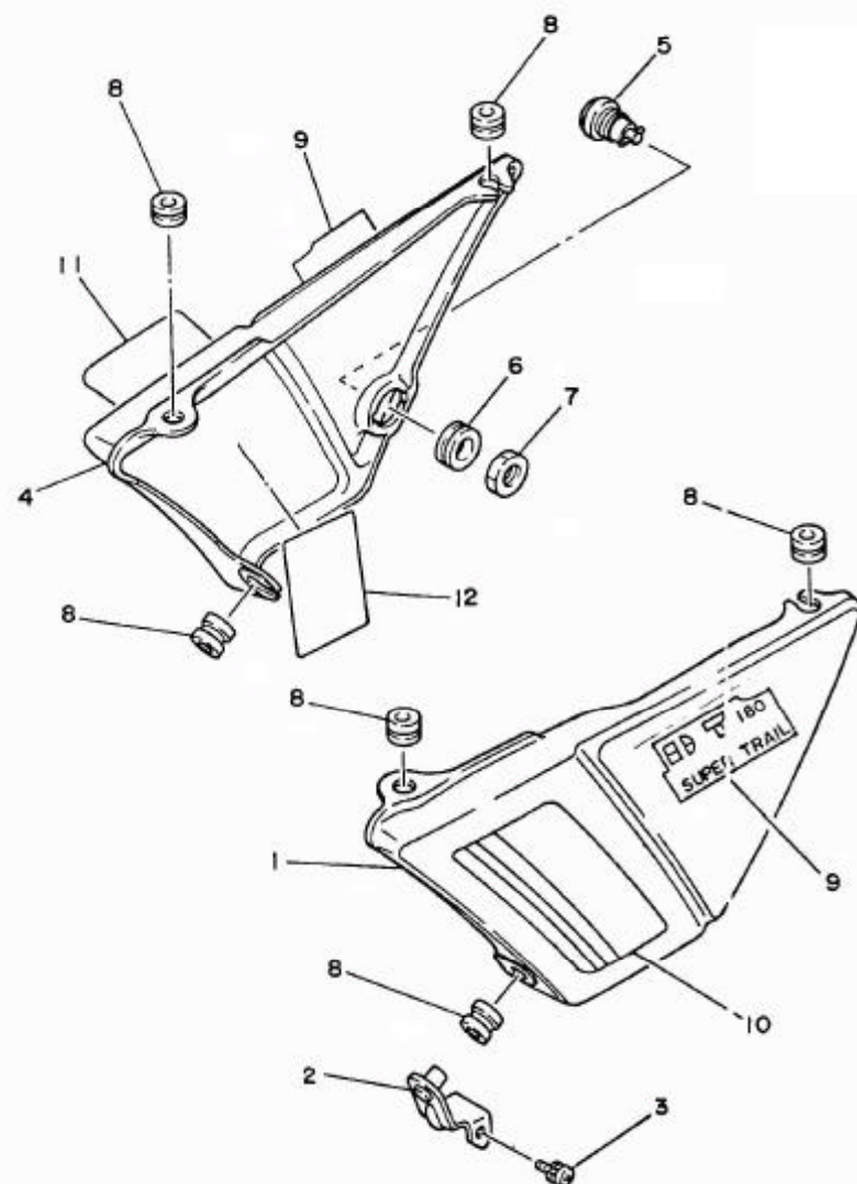
FIG. 19 TAMPAS LATERAIS
