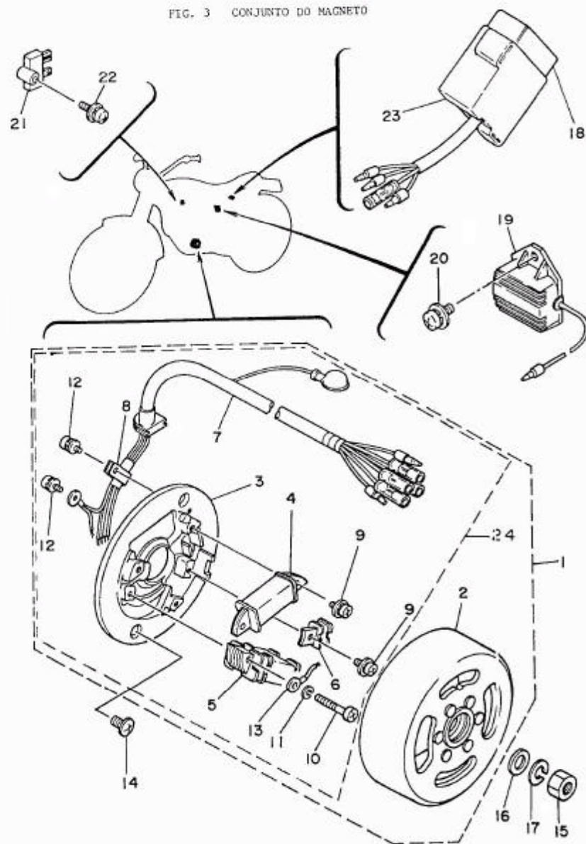
FIG. 3 CONJUNTO DO MAGNETO
