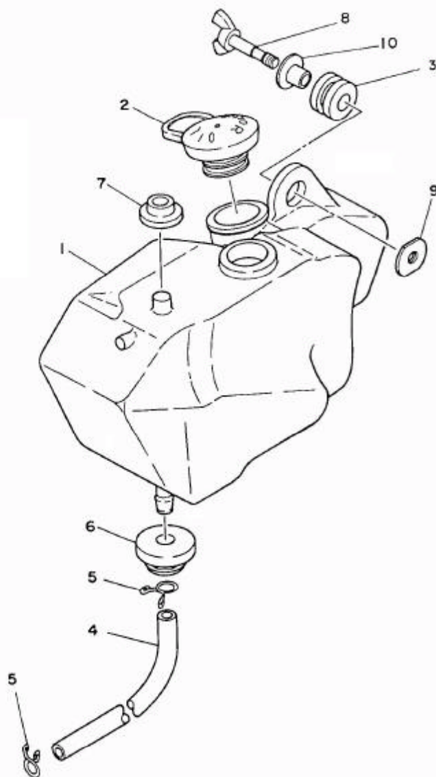
FIG. 20 TANQUE DE ÓLEO
