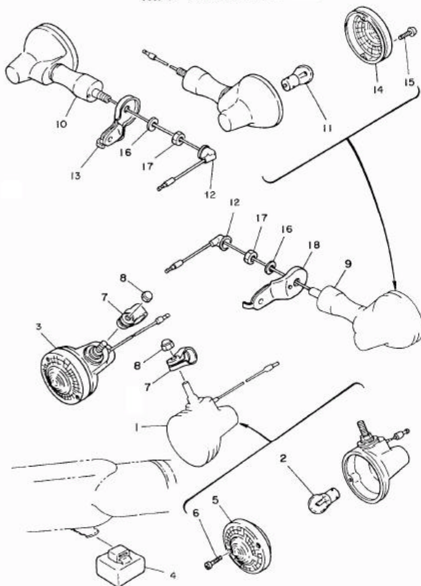
FIG. 31 SINALIZADORES(PISCA-PISCA)
