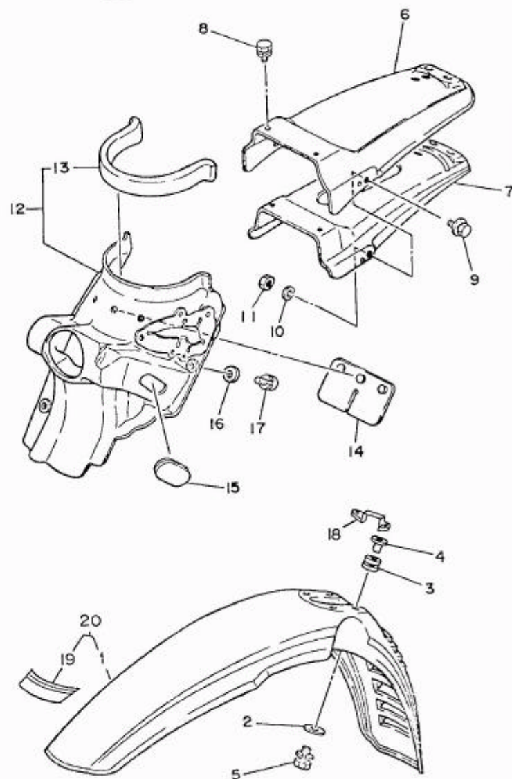
FIG. 18 PARALAMA DIANTEIRO E TRASEIRO
