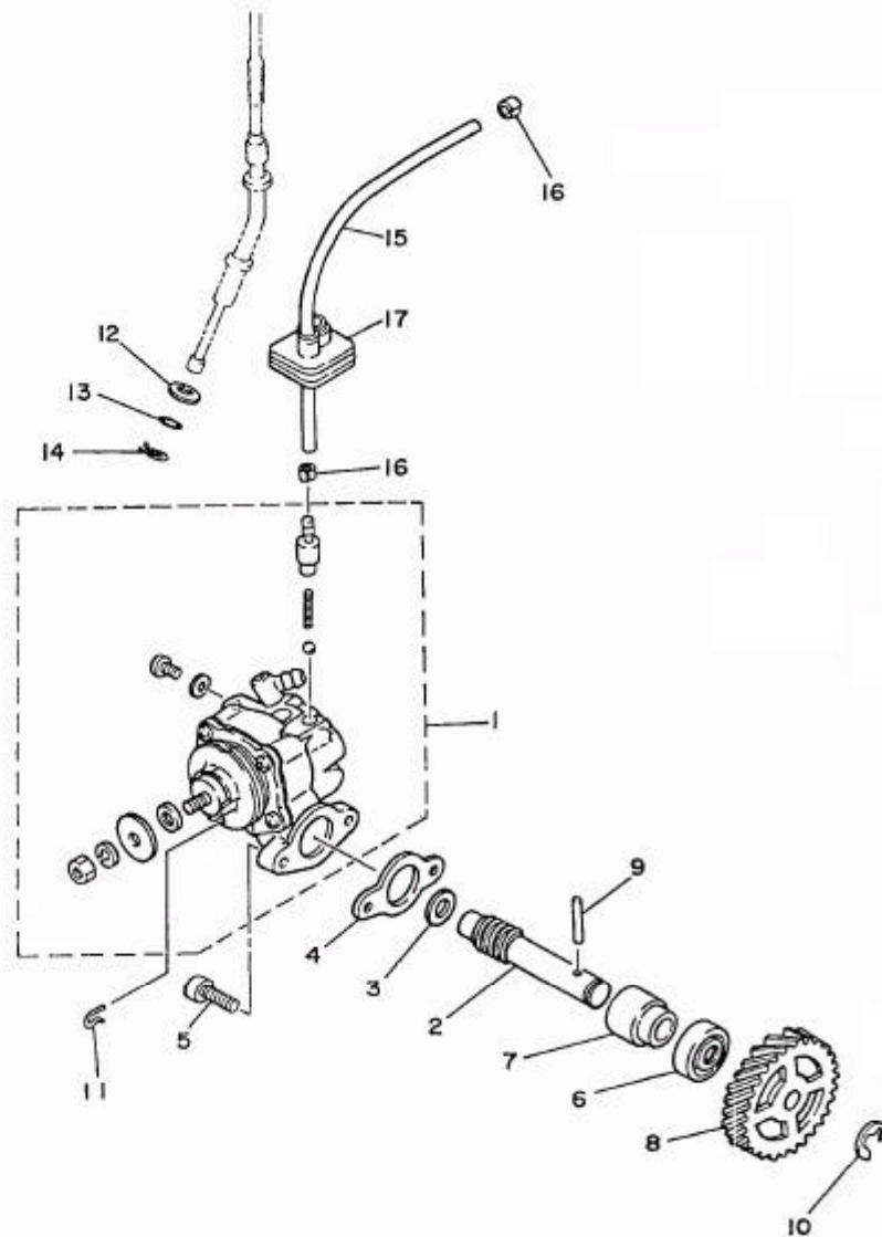
FIG. 4 BOMBA DE ÓLEO
