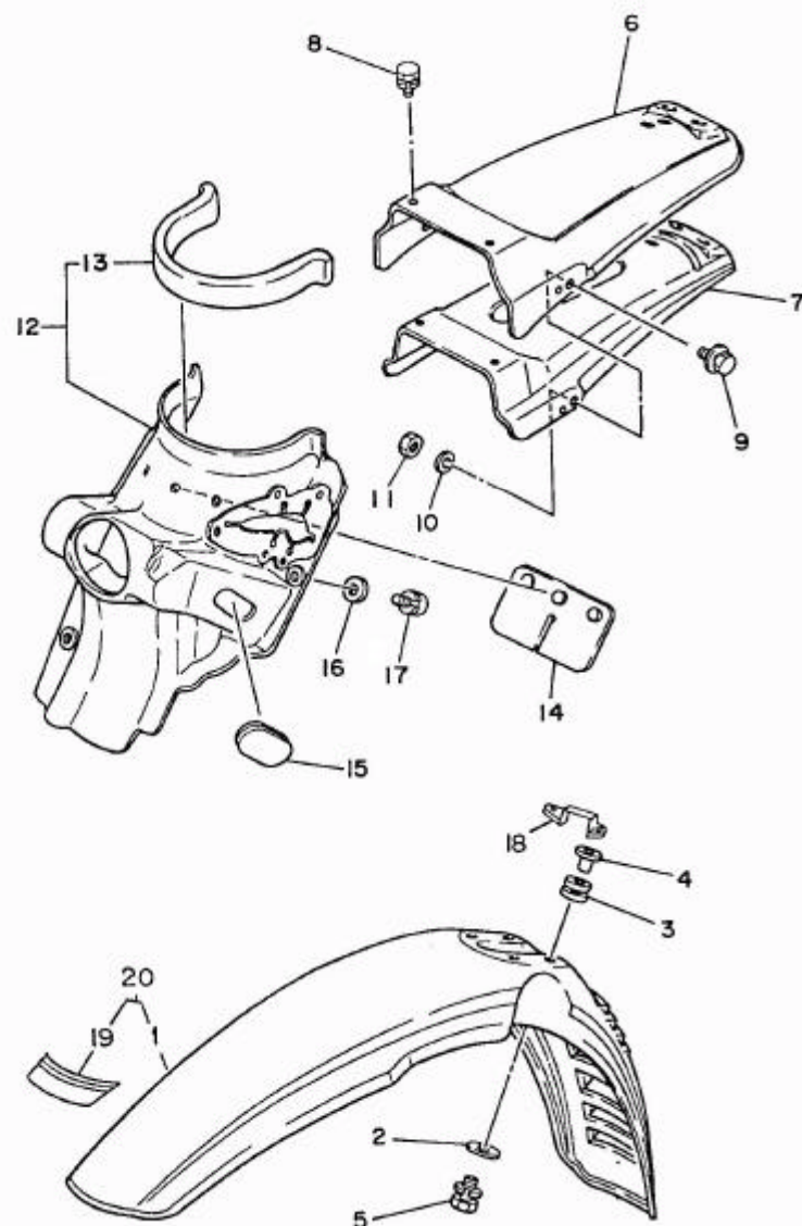
FIG. 18 PARALAMA DIANTEIRO E TRASEIRO
