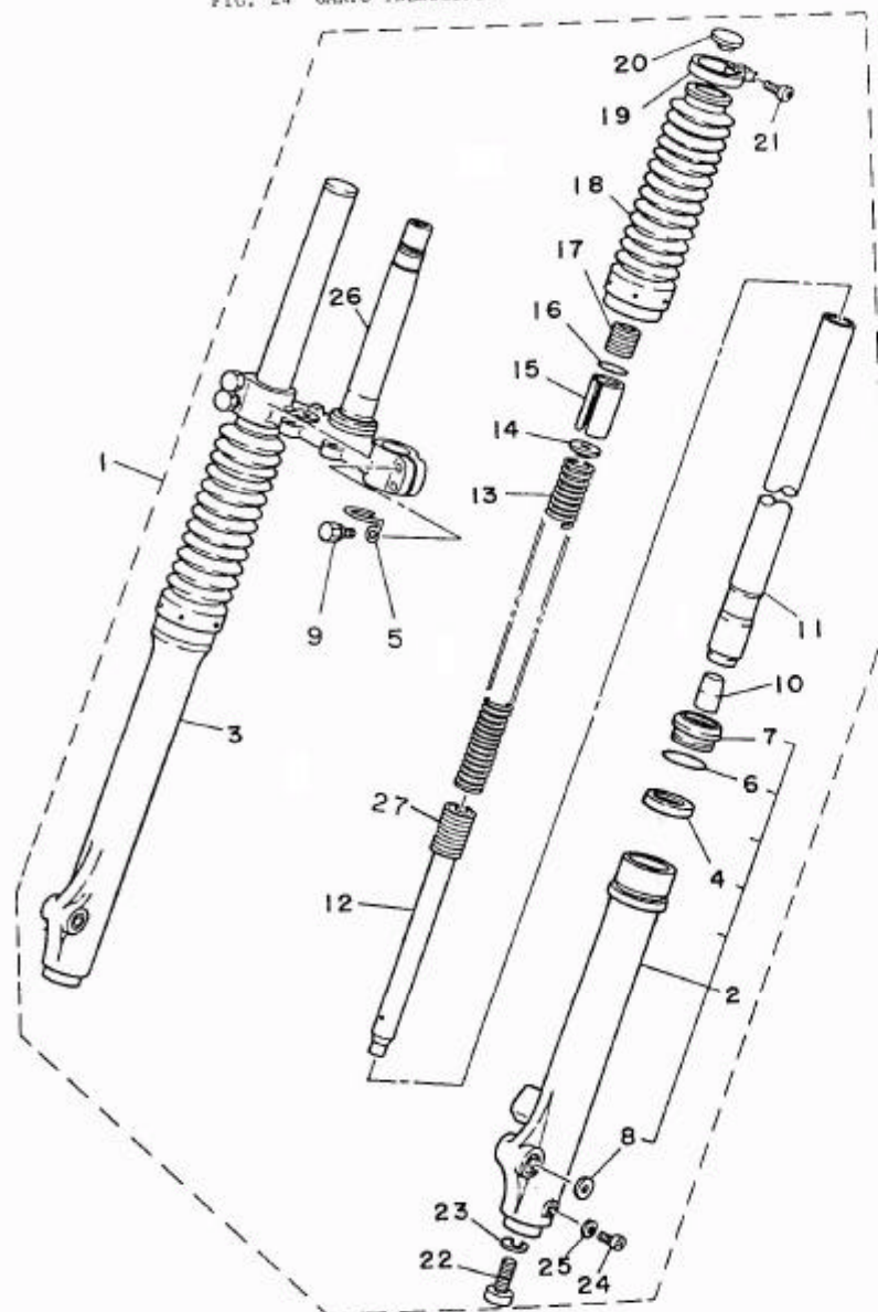
FIG. 24 - GARFO TELESCÓPICO
