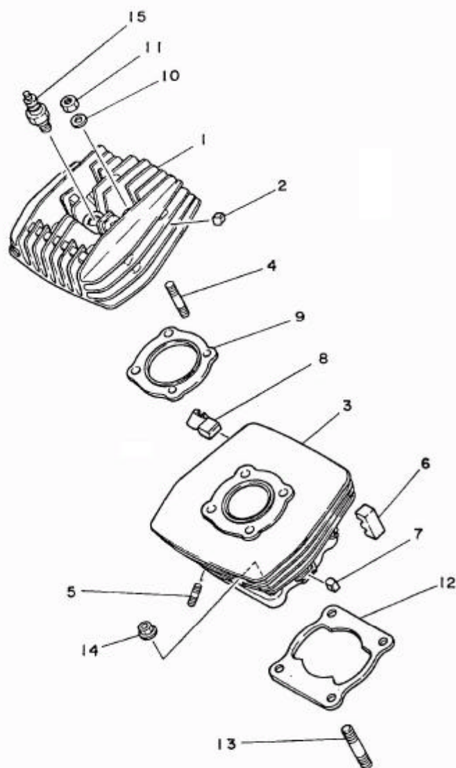
FIG. 1 CABEÇOTE E CILINDRO
