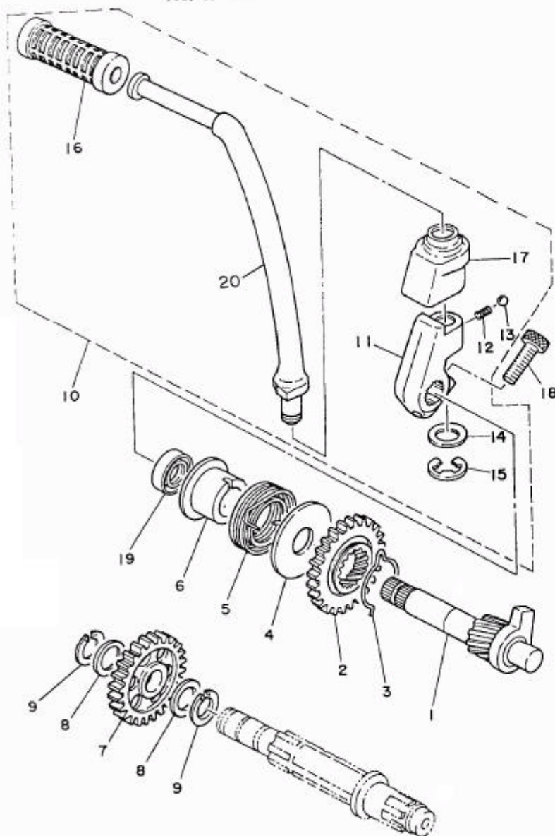
FIG. 11 EIXO E PEDAL DE PARTIDA
