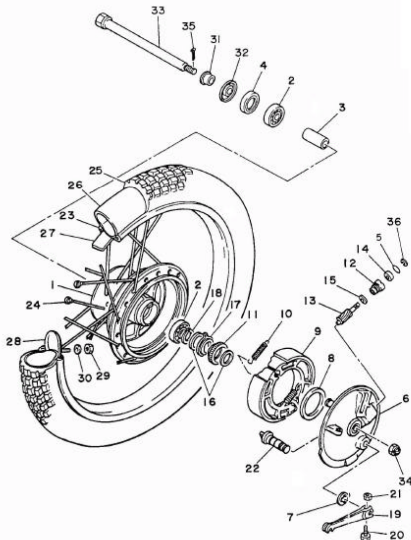
FIG. 27 RODA DIANTEIRA
