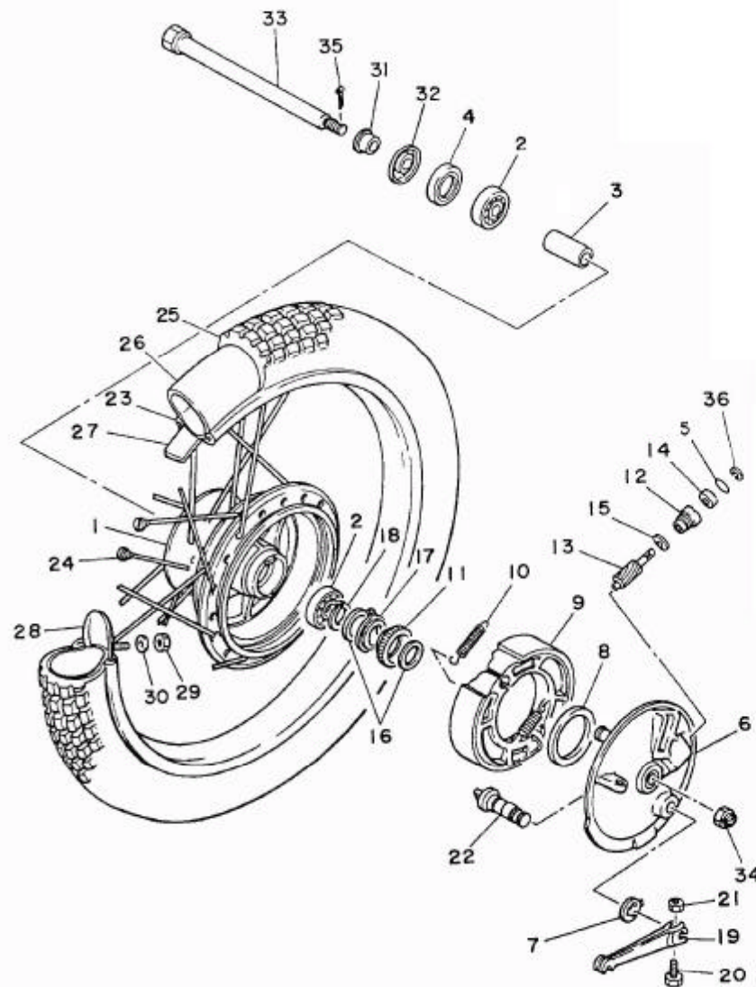
FIG. 27 RODA DIANTEIRA
