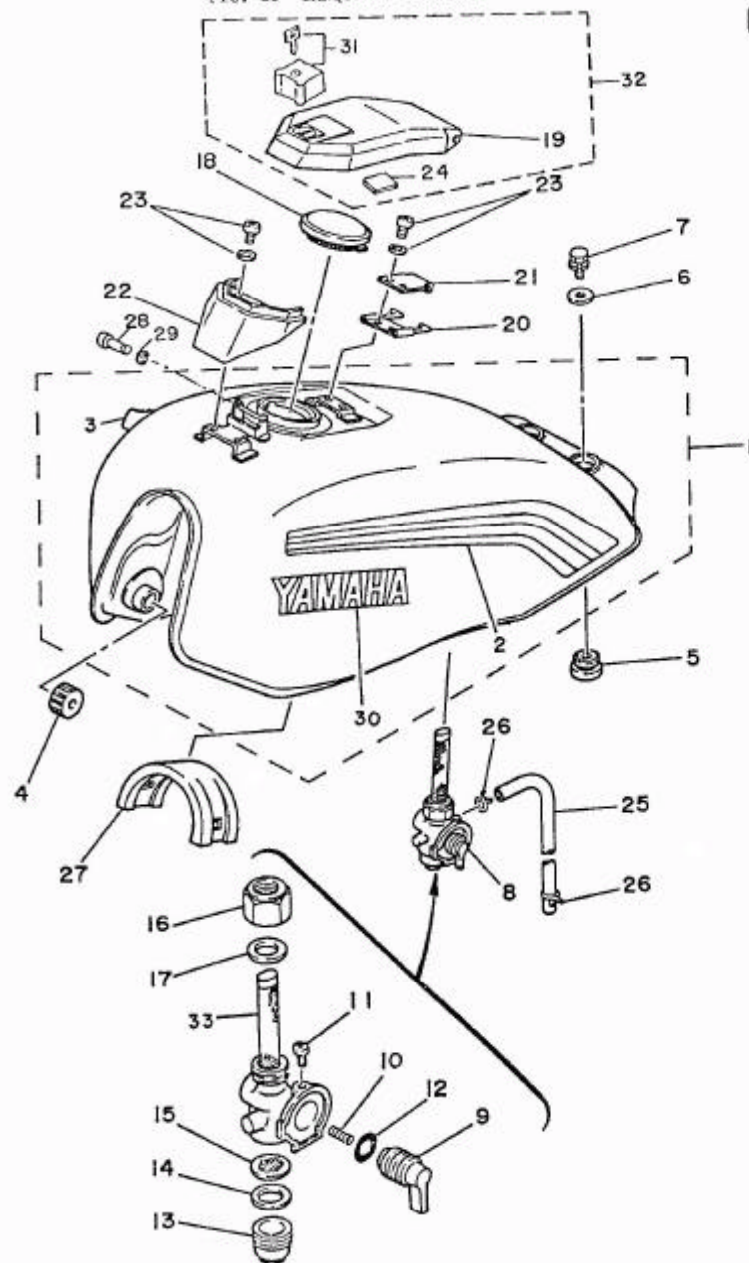
FIG. 25 TANQUE DE GASOLINA
