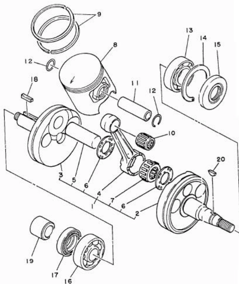
FIG. 2 VIRABREQUIM E PISTÃO
