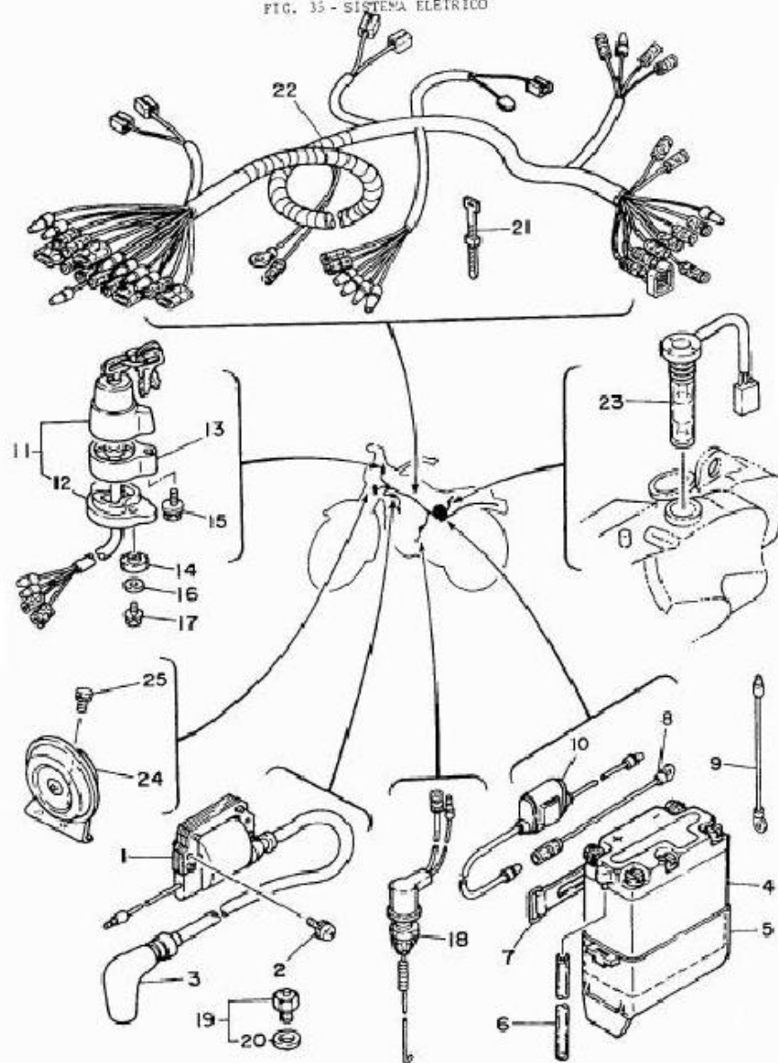
FIG. 35 - SISTEMA ELÉTRICO
