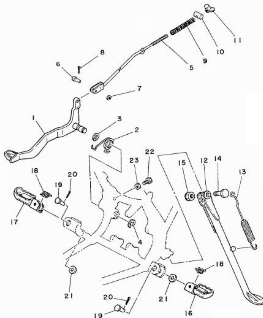
FIG. 30 CAVALETE DE ESTACIONAMENTO ESTRIBO DIANTEIRO E PEDAL DE FREIO
