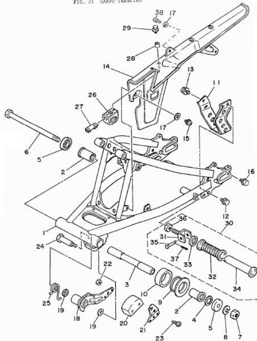
FIG. 21 GARFO TRASEIRO
