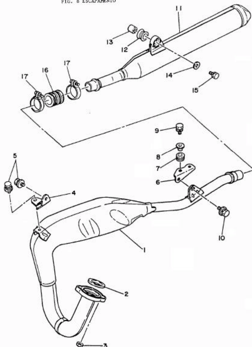
FIG. 8 ESCAPAMENTO
