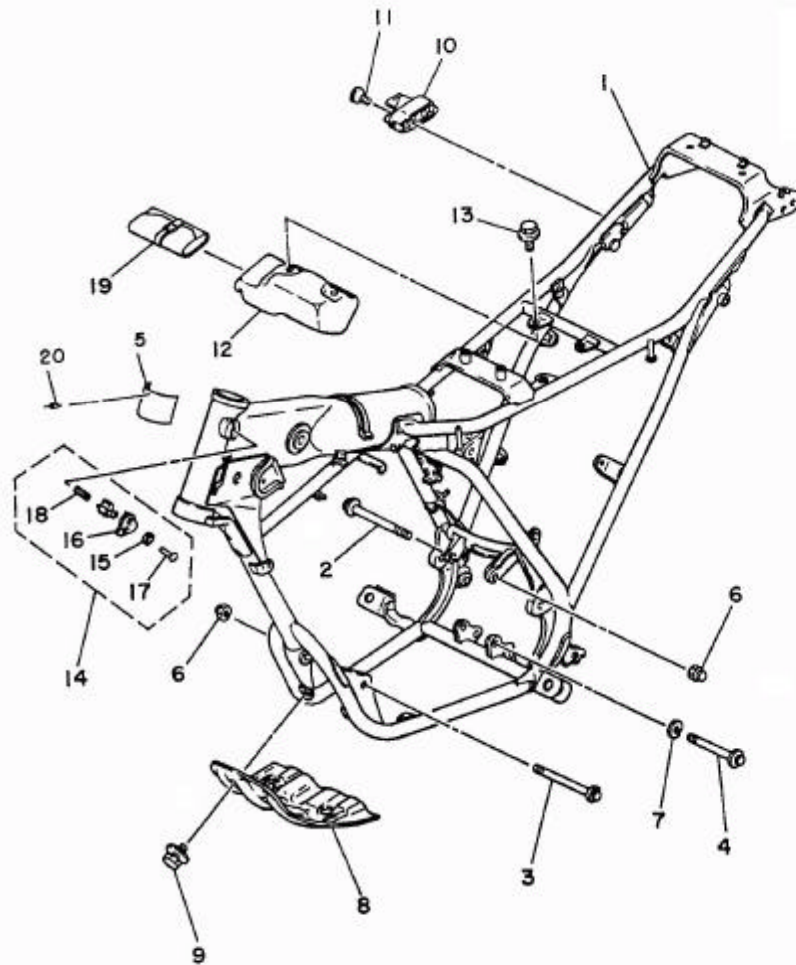
FIG. 17 CHASSI
