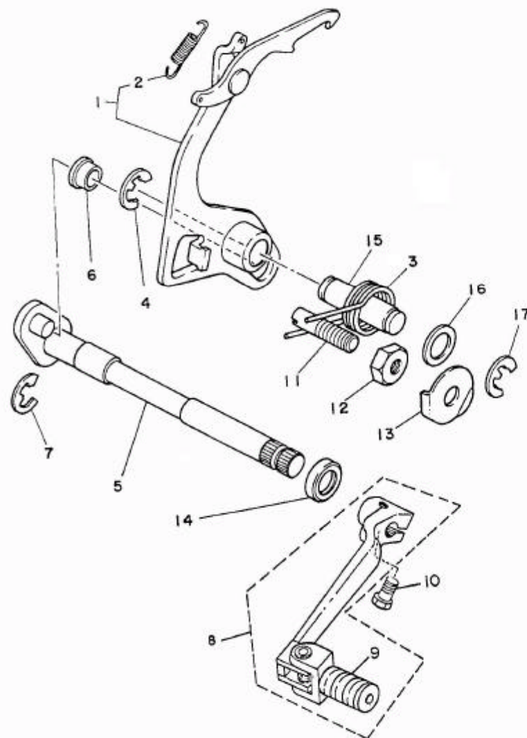
FIG. 16 EIXO E PEDAL DE CÂMBIO
