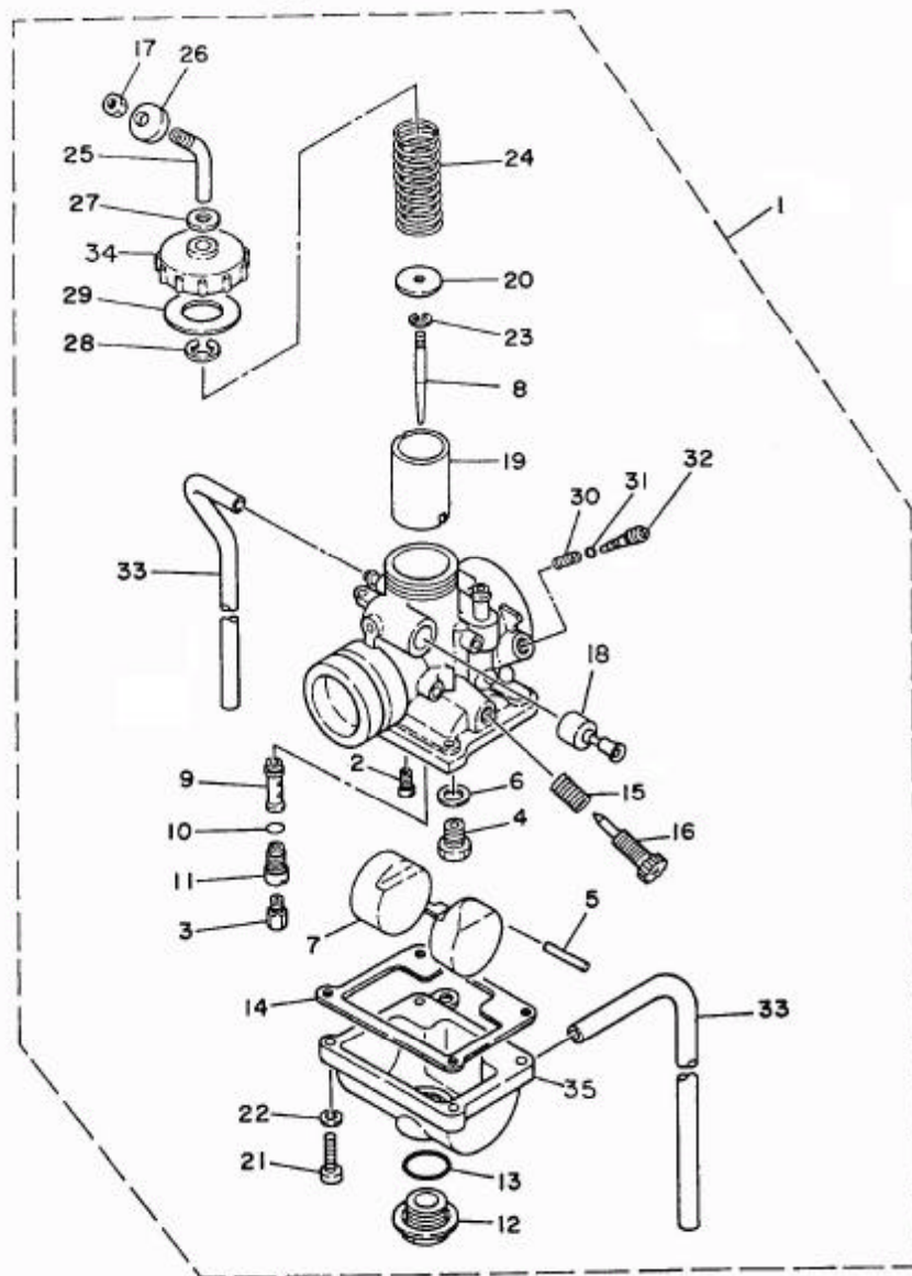
FIG. 7 CARBURADOR
