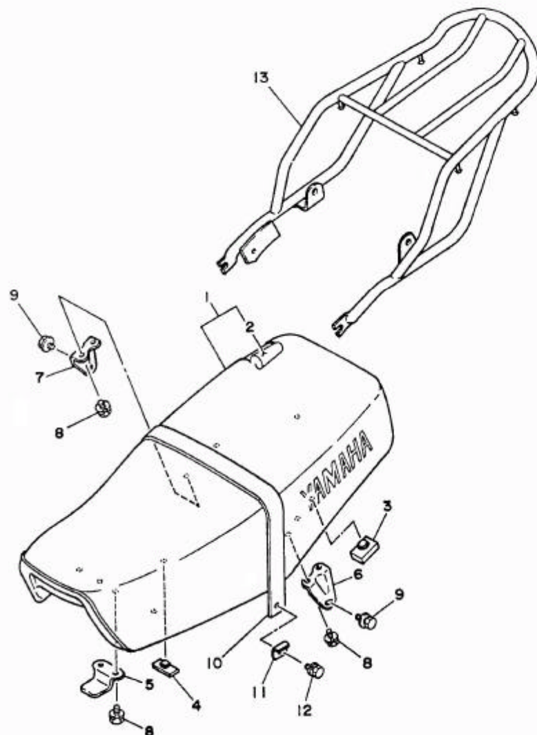
FIG. 26 ASSENTO
