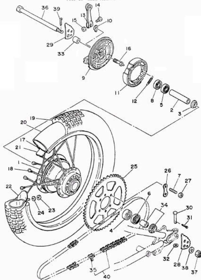
FIG. 18 RODA TRASEIRA
