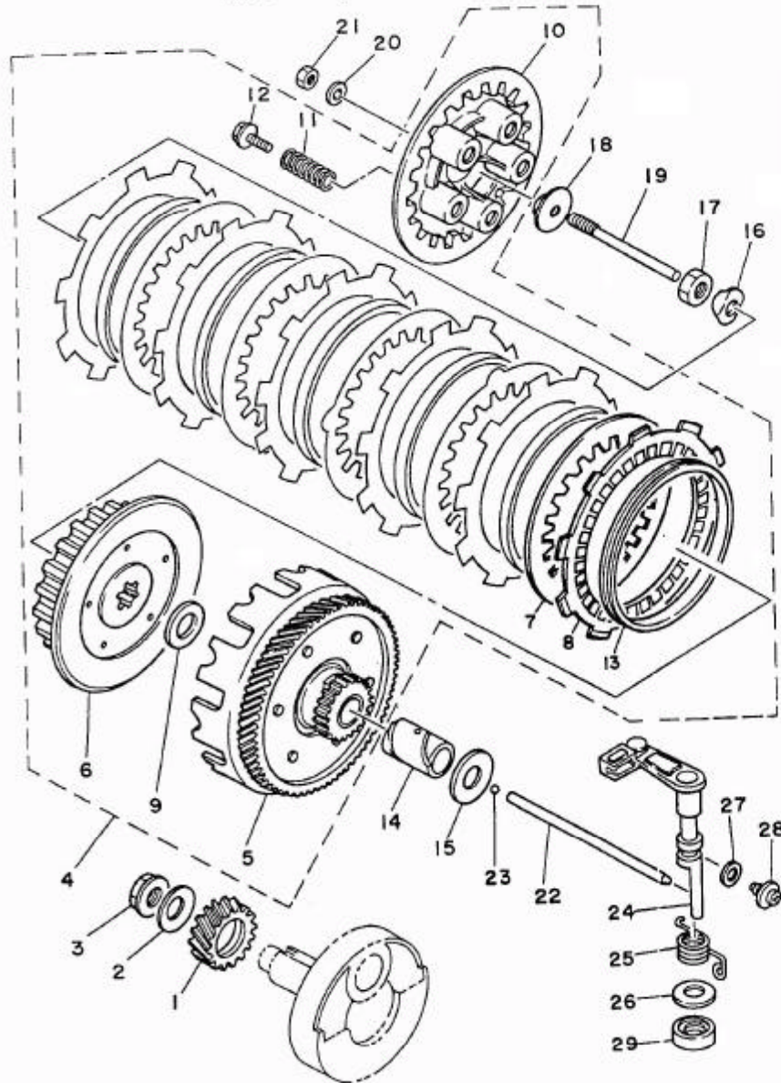
FIG. 12 - FRICÇÃO
