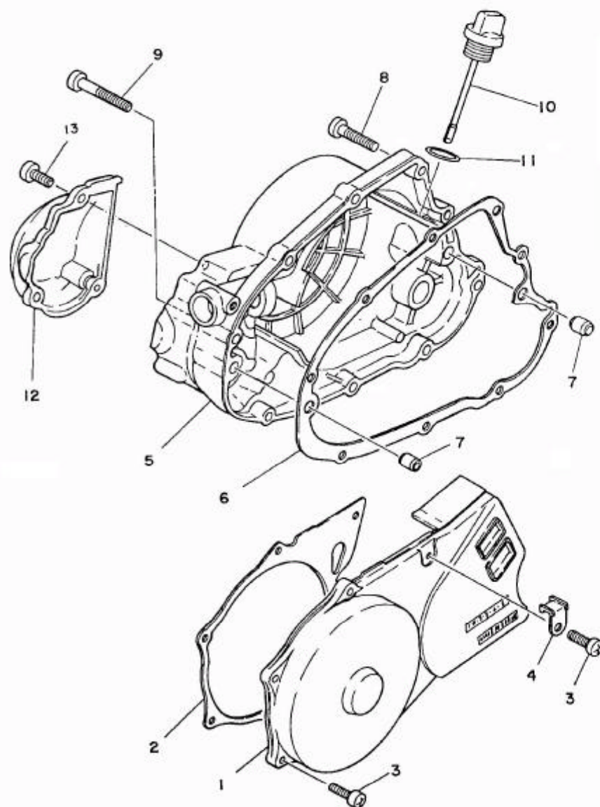
FIG. 10 TAMPAS DA CARÇAÇA
