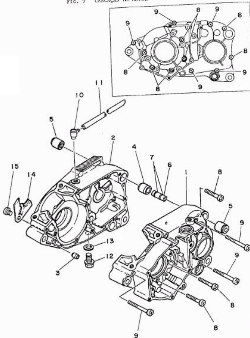
FIG. 9 CARCAÇAS DO MOTOR
